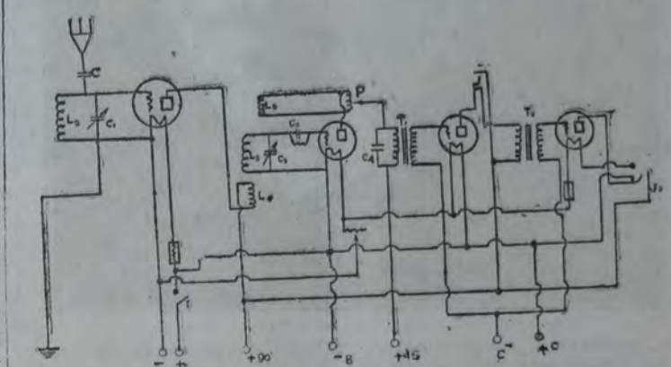
ESTE ES EL ESQUEMA REPRESENTATIVO DEL CIRCUITO DE gran alcance y selectividad que presenta el experto profesional F. LACONCA. Sus excelentes condiciones de funcionamiento nos lo hacen recomendar especialmente.
